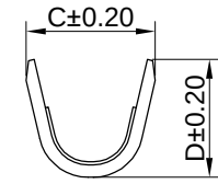
SEC:B-B
