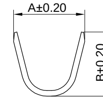
SEC:A-A
