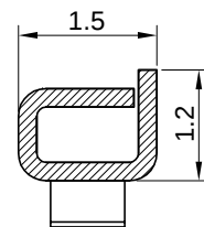
SEC:D-D
