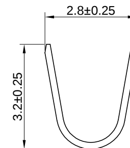
SEC:A-A
