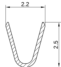
SEC:A-A
